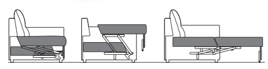
Schemat rozkładania funkcji spania typ. PUMA
